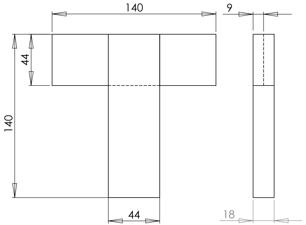
END ELEVATION
