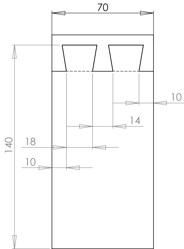
END ELEVATION
