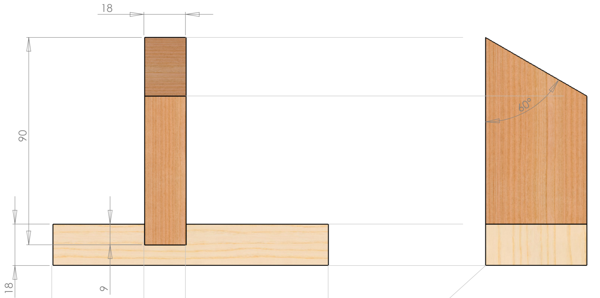
ELEVATION
